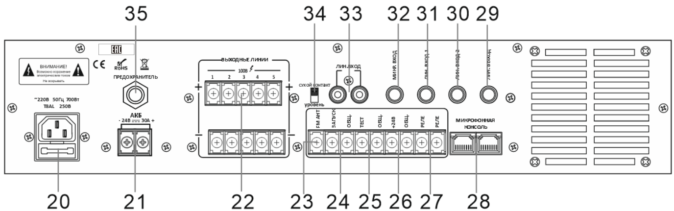
Рис. 1.3. Задняя панель
