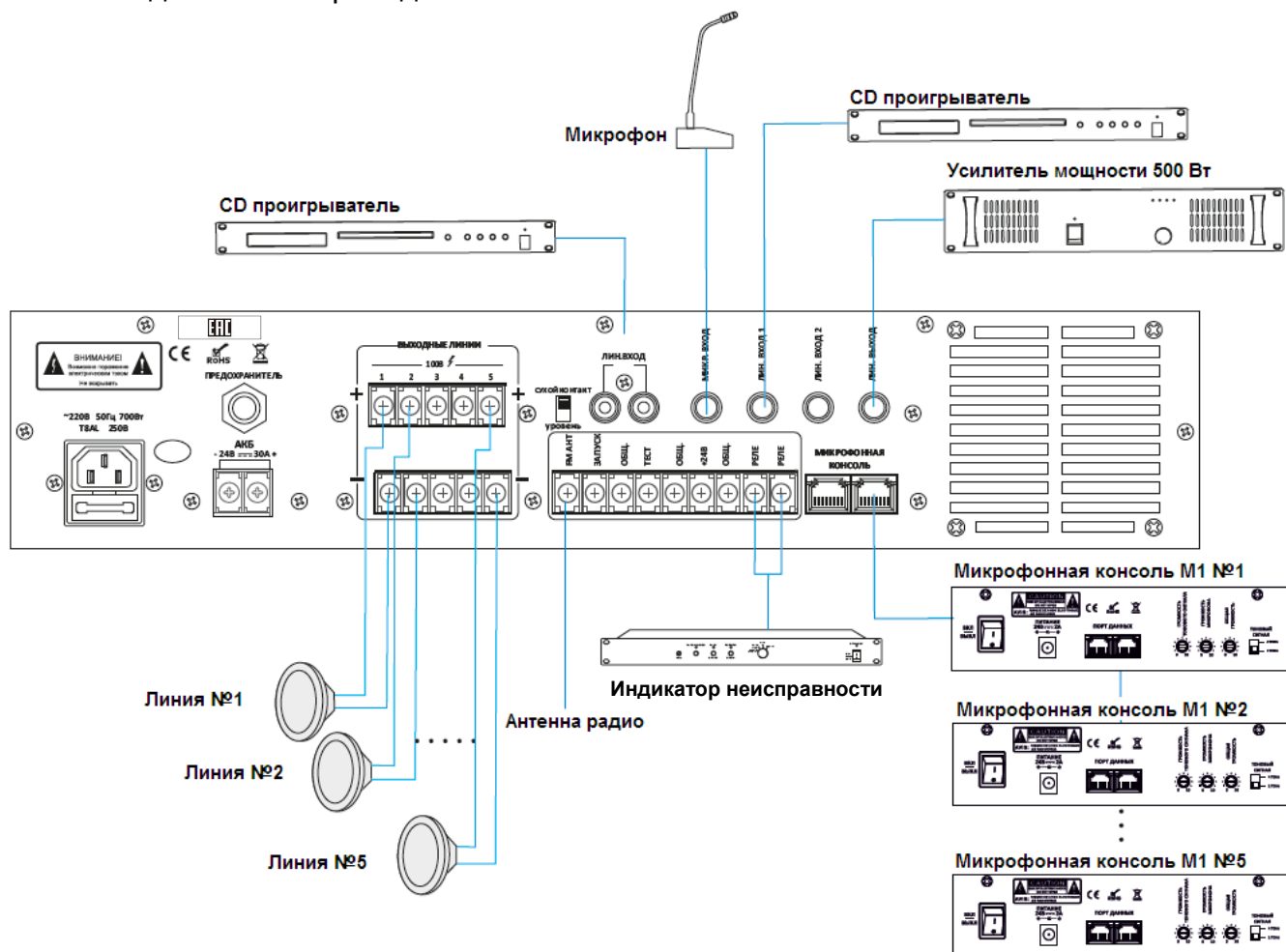
Рис. 2.1 Схема подключения
