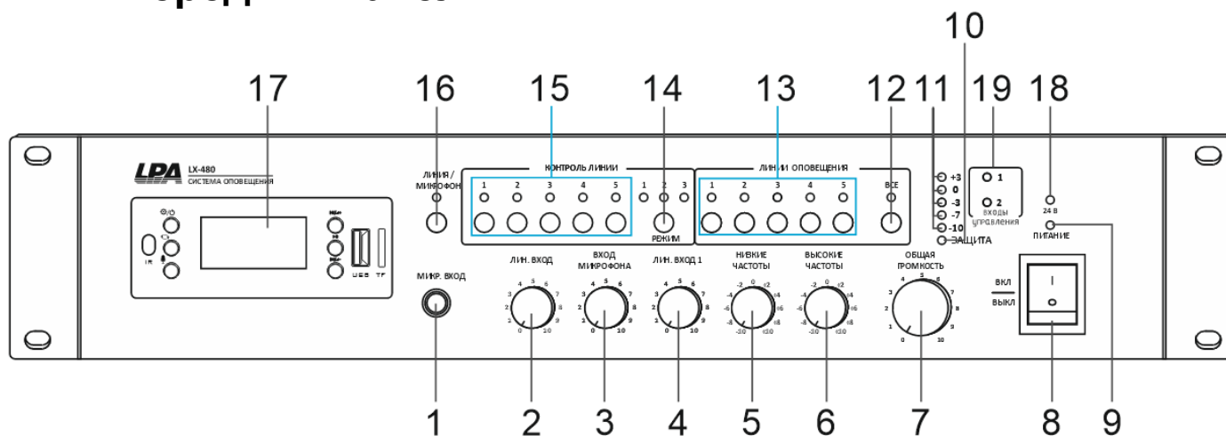
Передняя панель
